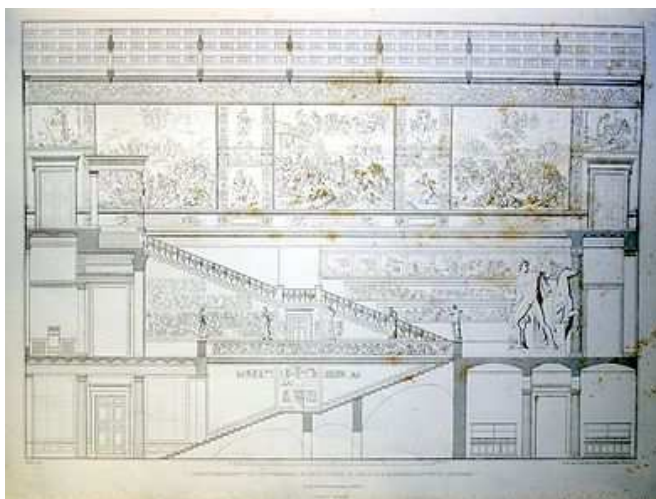
Längsschnitt, Treppenhaus mit Wandgliederung, Riedel 1862
